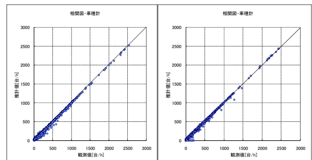
図-3 推定交通量と観測交通量の散布図(2008/4/1)
