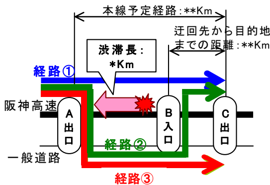
図-2 障害渋滞時迂回経路選択の概要
