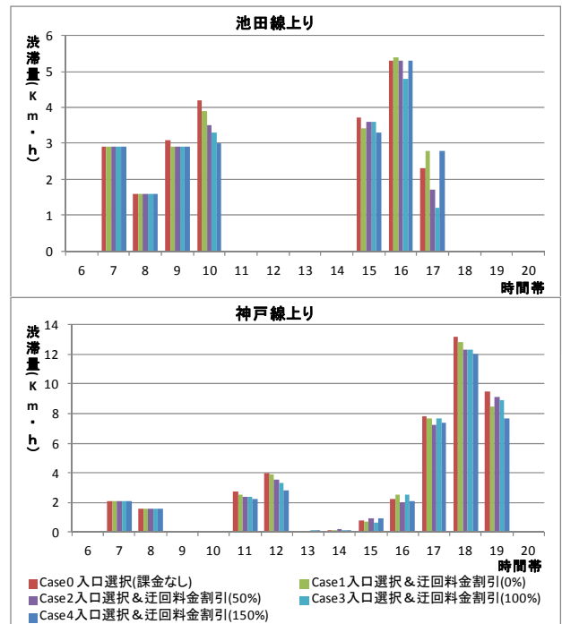
図-5 流出制御実施時の時間帯別渋滞量の比較
