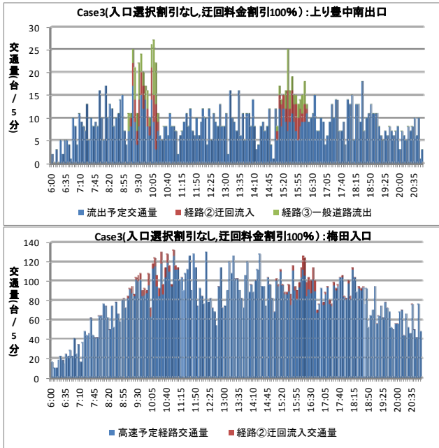
図-4 迂回経路の出入口交通量(上：出口, 下：(再)流入) [Case3, 迂回料金割引100%, 池田線]
