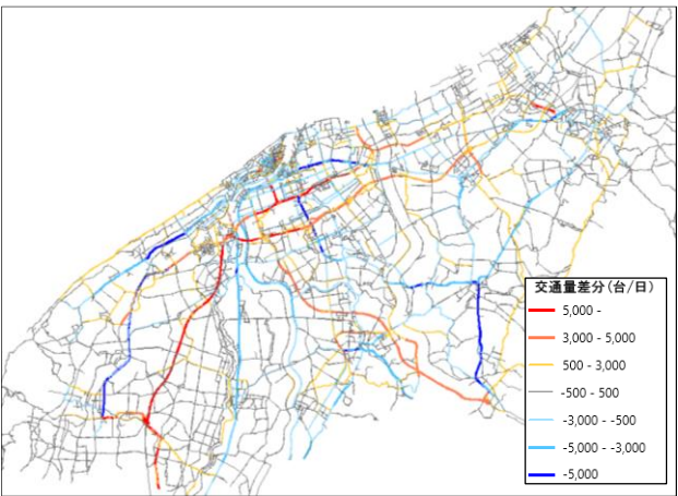
図 4-2 交通量差分図 (ケース 5ーケース 1)
